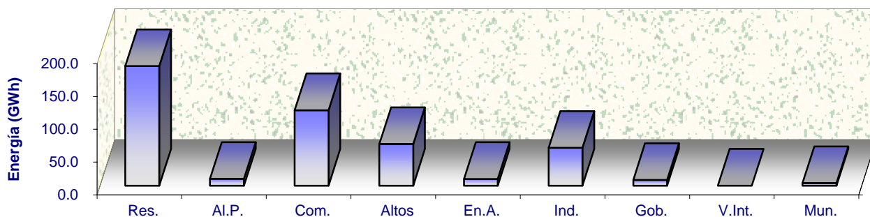
ENERGIA VENDIDA POR SECTORES DE CONSUMO AGOSTO 2008
