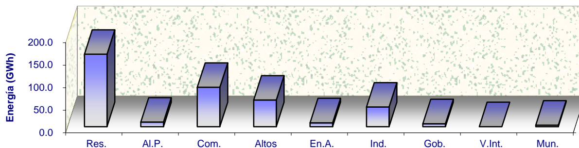
ENERGIA VENDIDA POR SECTORES DE CONSUMO DICIEMBRE 2008
