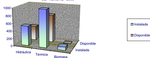
CAPACIDAD INSTALADA Y DISPONIBILIDAD EN PLANTAS SEPTIEMBRE 2009
