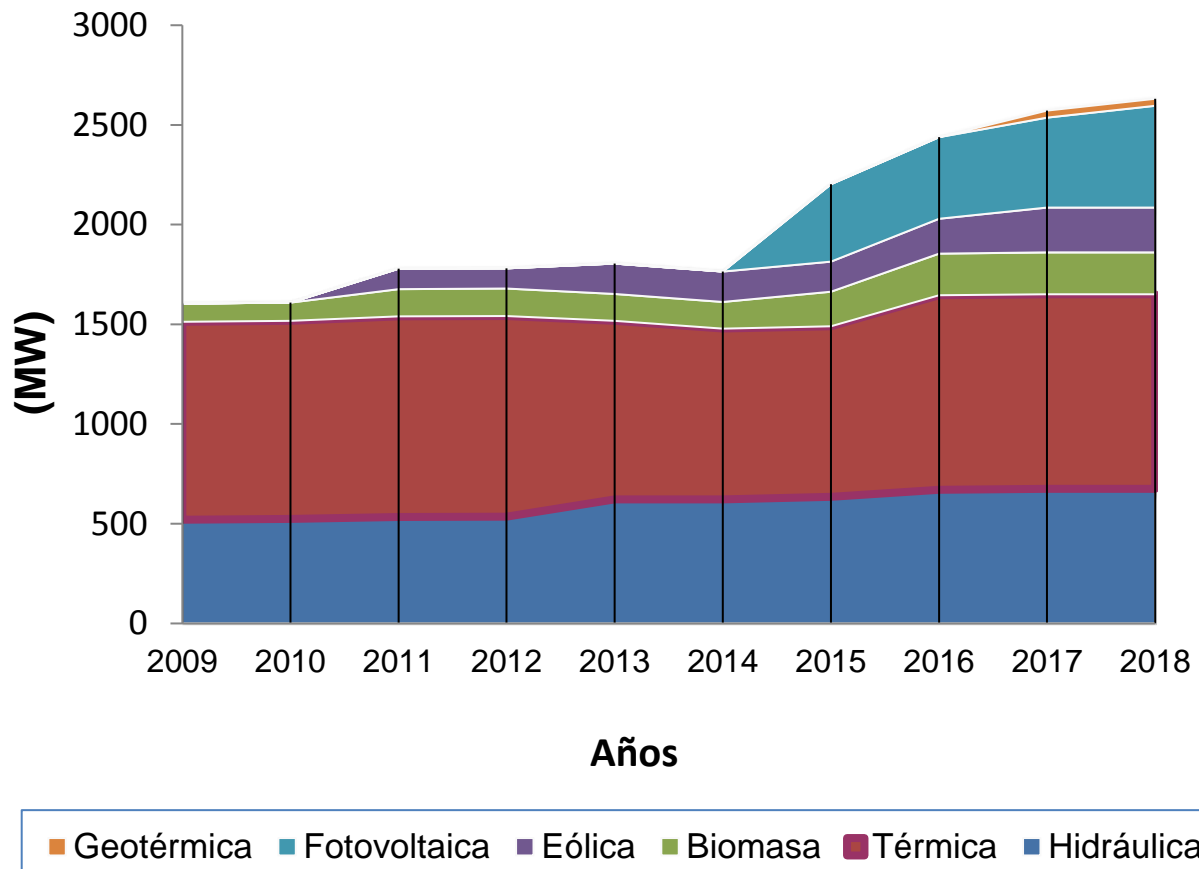
Gráfica No.1 Capacidad Total Instalada 2009-2018
